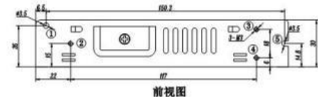
前视图
